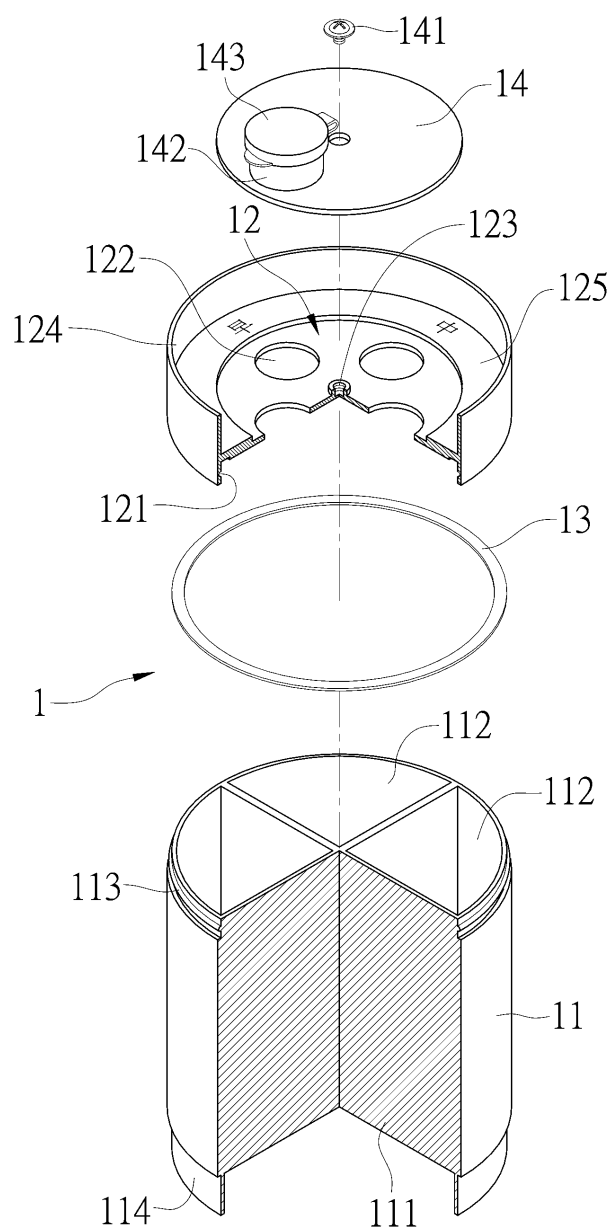
第十圖：本創作之又一使用狀態立體旋出結構示意圖
